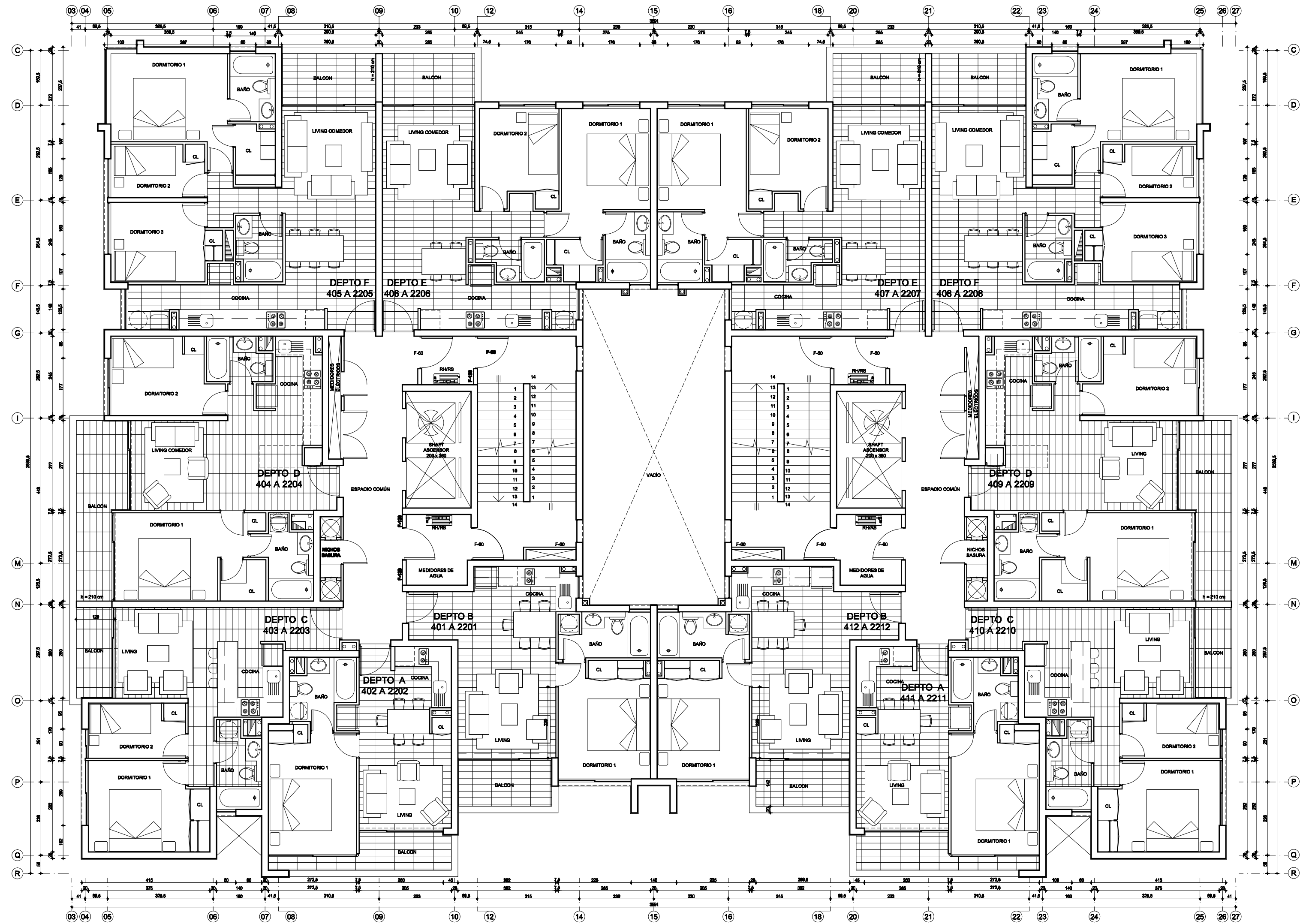
PLANTA 4° - 22° PISO 1:100
