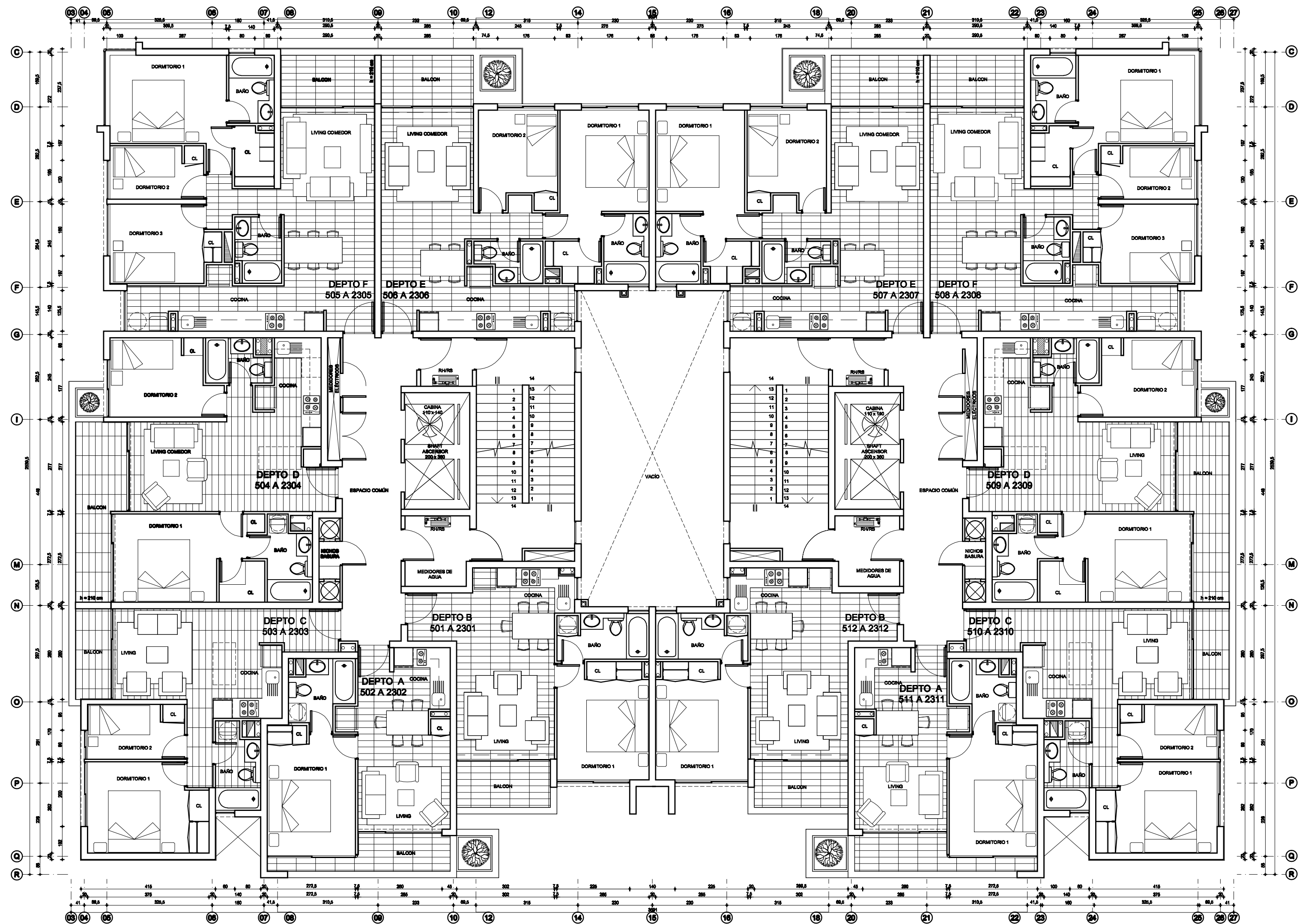
PLANTA 5° - 23° PISO 1:100
