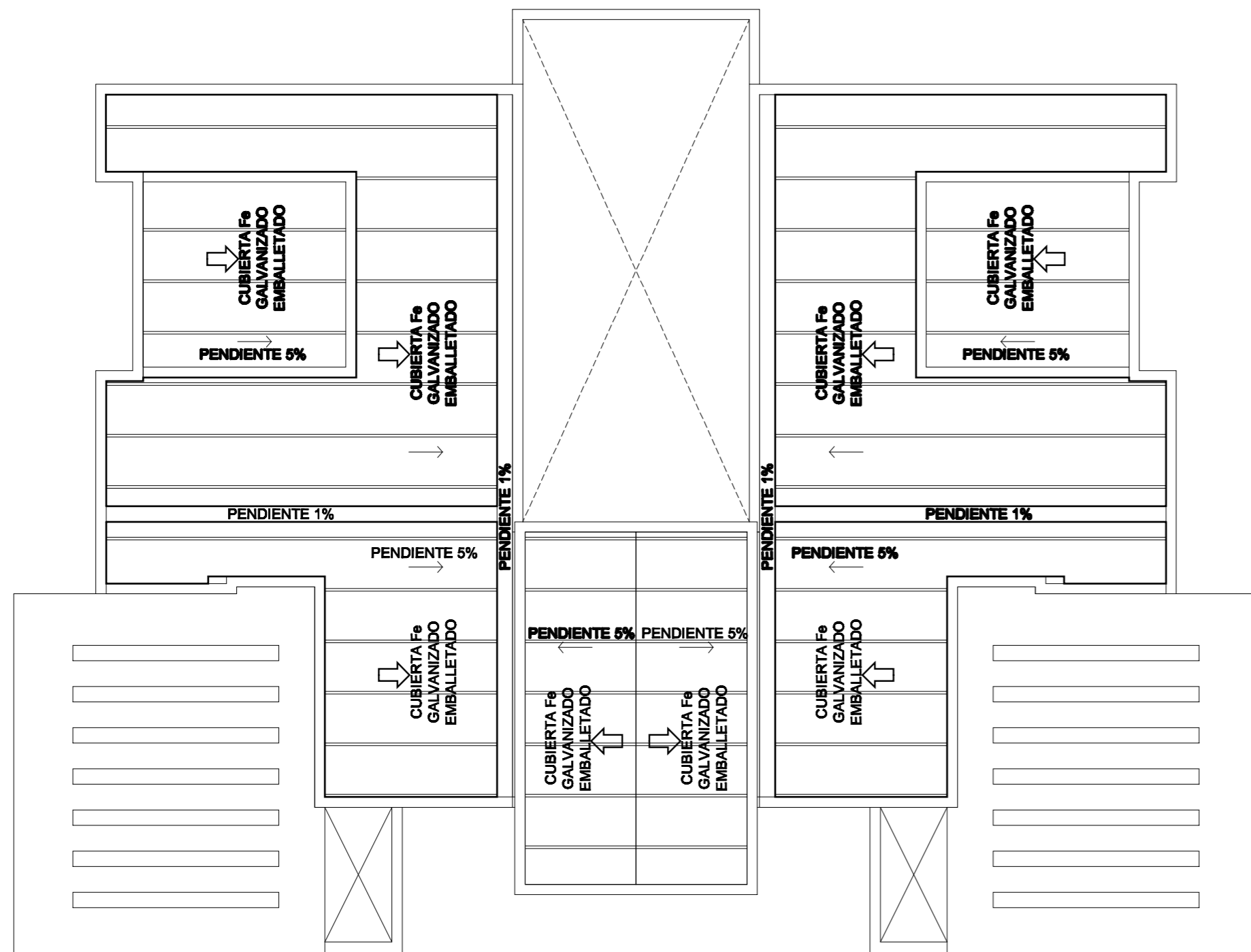
PLANTA CUBIERTA 1:100
